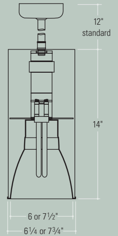
PENDANT MOUNT
