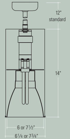
PENDANT MOUNT
